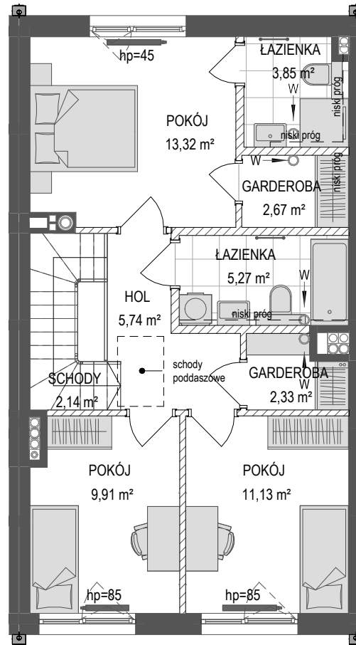
PIĘTRO 1 56,36 m 2
